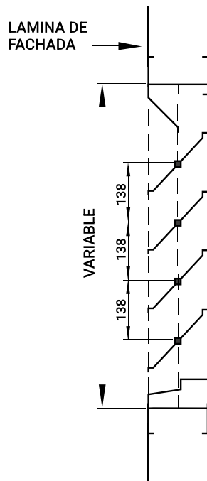
INSTALACIÓN EN FACHADA ESTRUCTURAL
