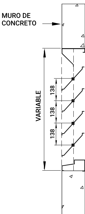
INSTALACIÓN EN MURO DE CONCRETO
